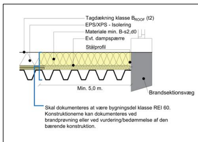
Figur 2.4 - Spring i bygningshøjde (høj/lav brandsmitte)
