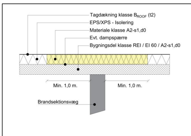
Figur 14.3 – Brandkamserstatning med brandbælte
