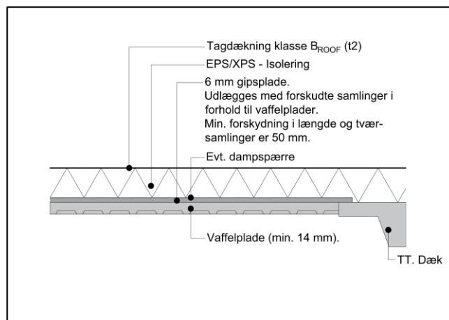
Figur 3.2 – Normalsnit (med gips)
