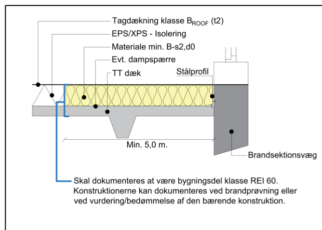
Figur 3.4 - Spring i bygningshøjde (høj/lav brandsmitte)
