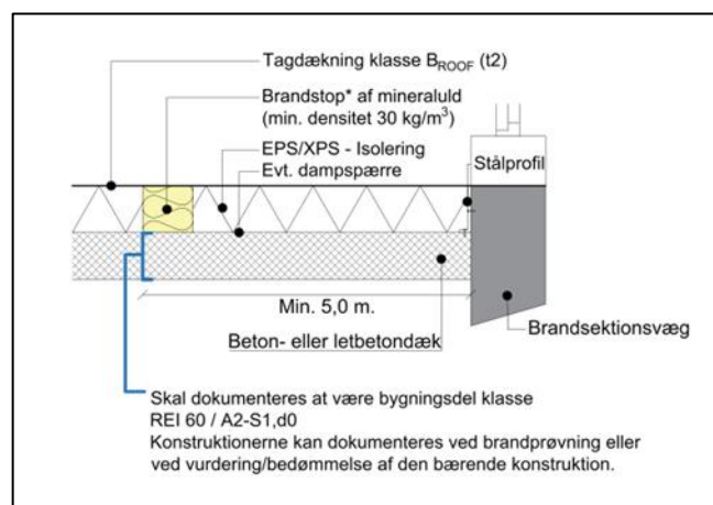
Figur 1.3 – Spring i bygningshøjde (høj/lav brandsmitte)
