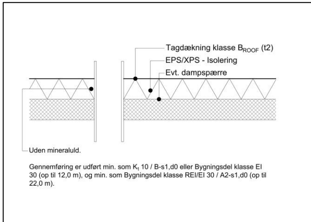
Figur 8.1 - Gennemføring uden behov for mineraluld
