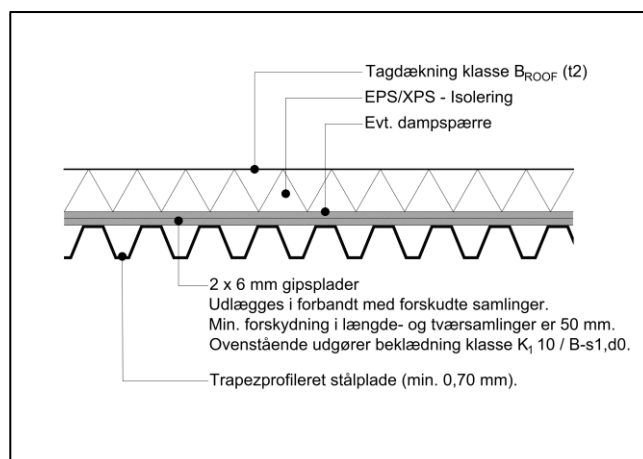
Figur 2.2 – Normalsnit (med gips)
