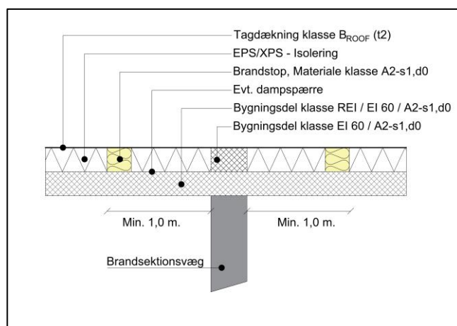
Figur 14.4 – Brandkamserstatning med brandstop
