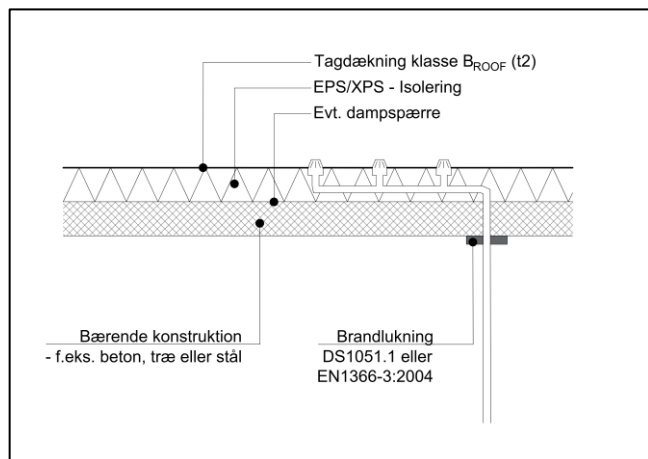
Figur 9.1 – Afvandingssystem (gennembrydning af dæk)
