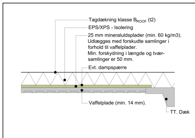
Figur 3.1 – Normalsnit (med mineraluld)
