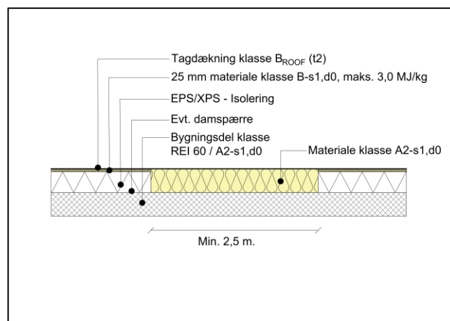
Figur 12.4 - Normalsnit tagopdeling med brandbælte
