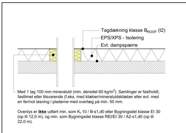
Figur 8.3 - Gennemføring med 1 lag mineraluld
