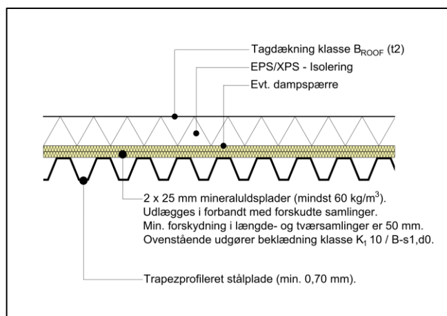
Figur 2.1 – Normalsnit (med mineraluld)
