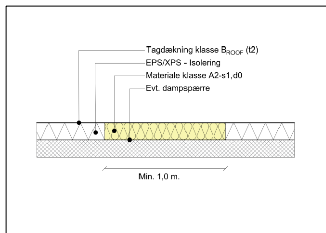
Figur 12.2 - Normalsnit tagopdeling med brandbælte
