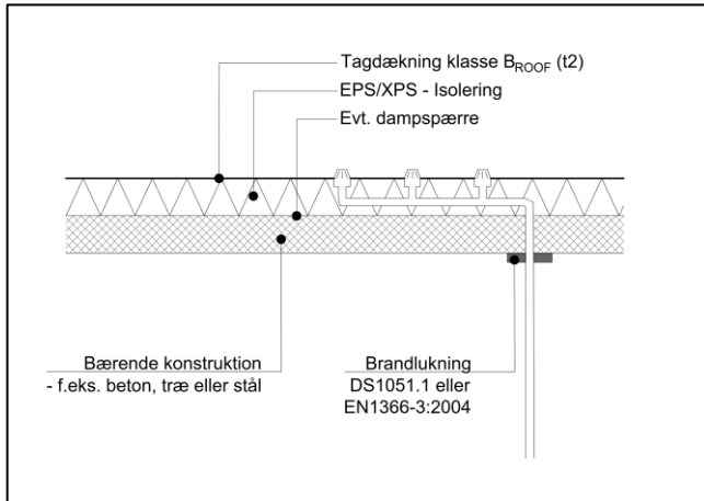
Figur 9.1 – Afvandingsystem (gennembrydning af dæk)
